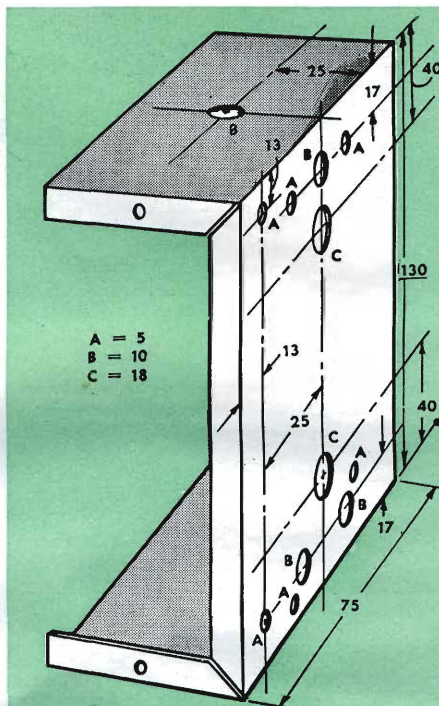
Fig. 2 - Telaio di alluminio. Le misure sono in millimetri
