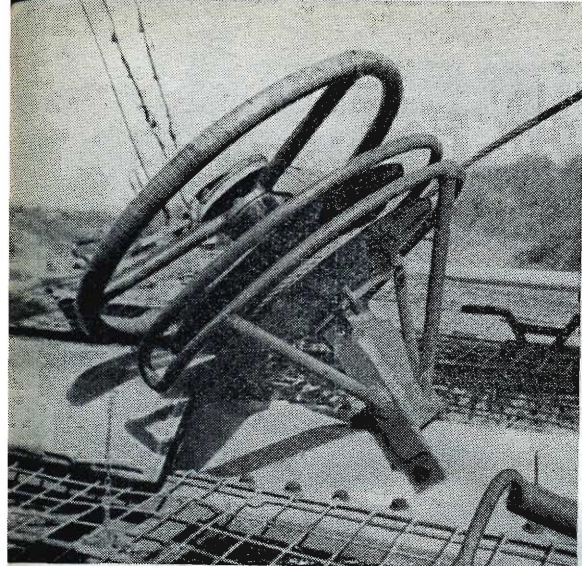
Sopra: situato nella parte anteriore dello yacht, il verricello a volante e il cavo tengono tesa la vela
