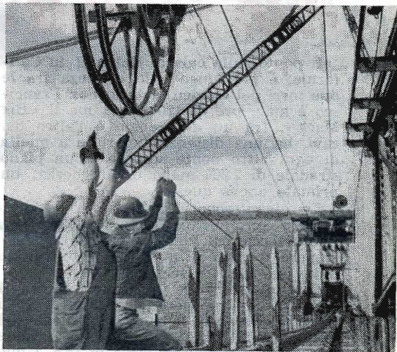
Il « filo morto » viene collocato nel cavo a mano a mano che la puleggia passa davanti agli operai
